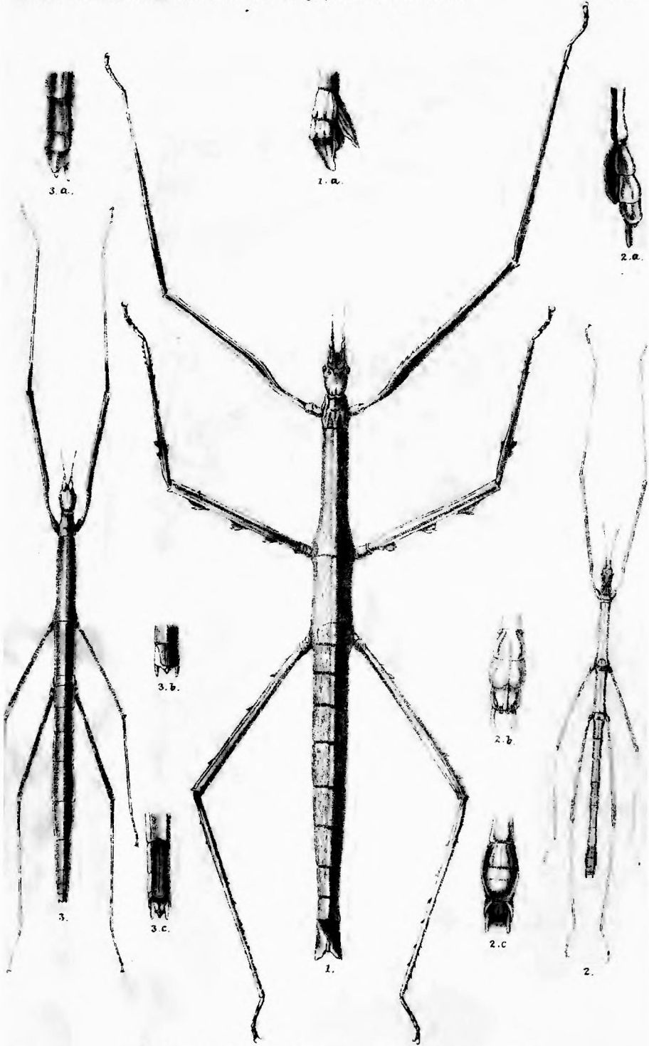
Fig. 1 B. scabriusculus , p. 55. Fig. 2-3 B. hispidulus , p. 47. For further explanation see p. 56.
