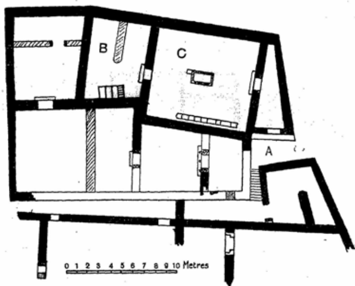
Fig. 51. House at Praesos.
