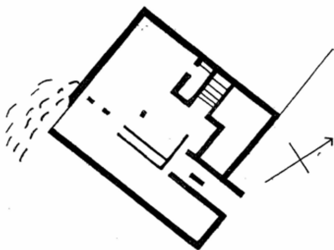
Fig. 13. House in Psira.
