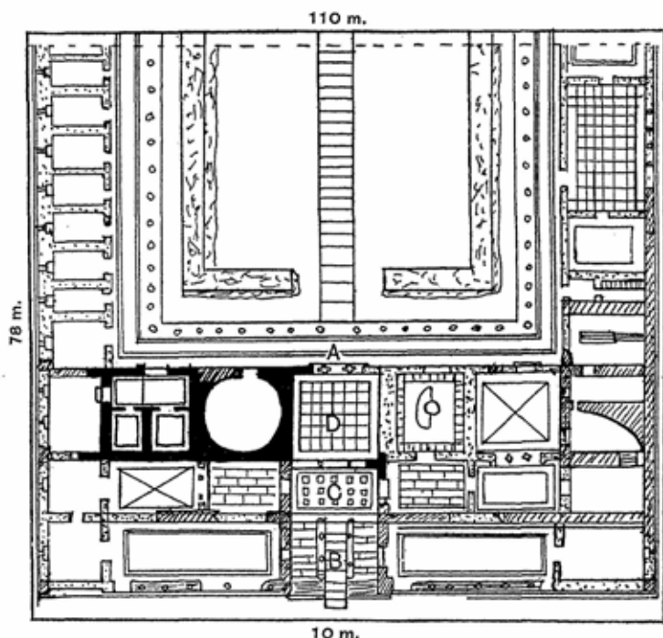
Fig. 39. Palace at Palatitza
