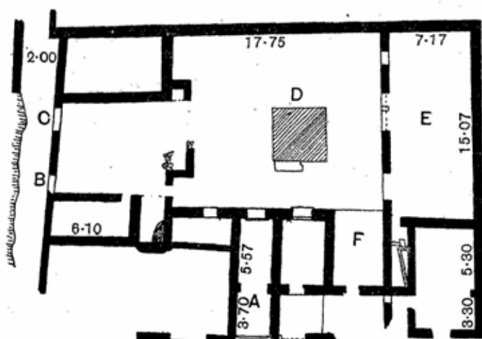
Fig. 50a. House at Delos.
