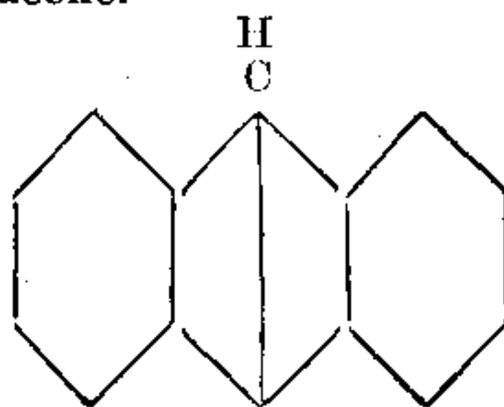
Anthracene.
