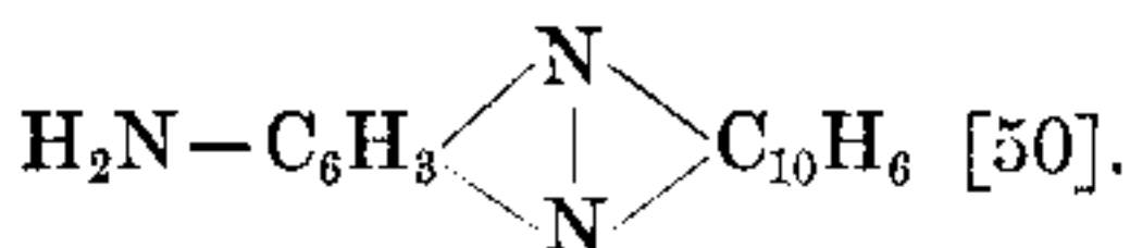
Eurhodine,
