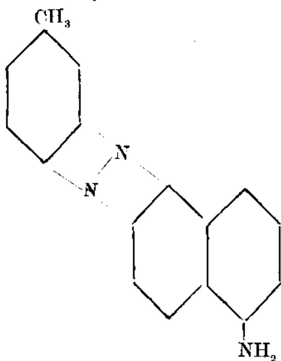
Eurhodine,
