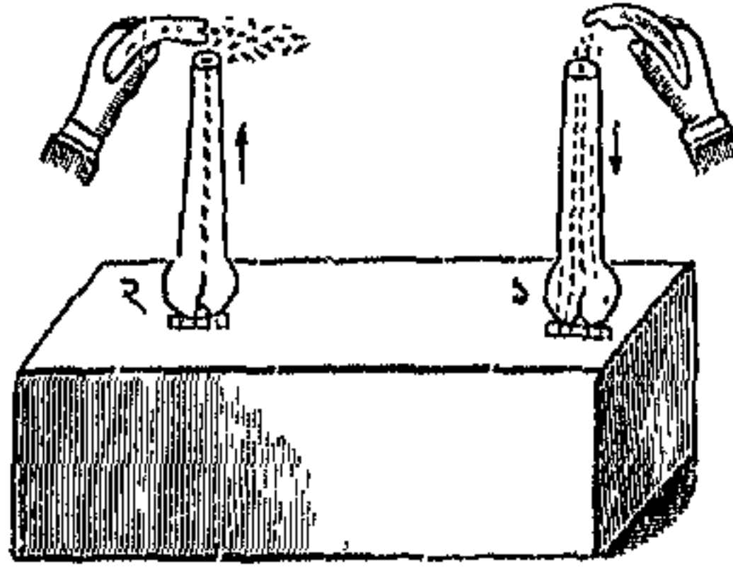
৭২ চিত্র ।—বায়ুর উর্দ্ধ ও নিম্নগতি ।
