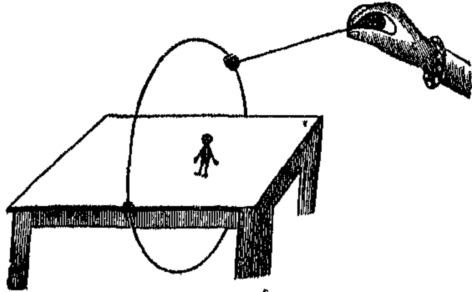
৭০ চিত্র ।—সূর্য্যের উদয়াস্ত ।
