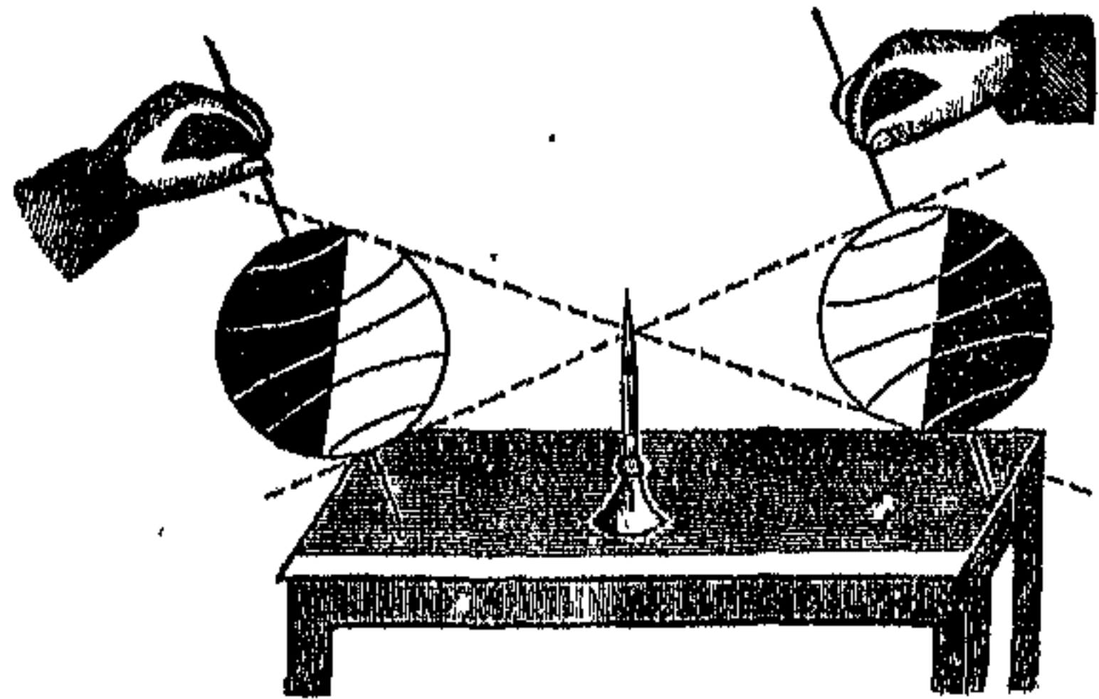
৭৯ চিত্র।—দিবা রাত্রির হ্রাস বৃদ্ধি।
