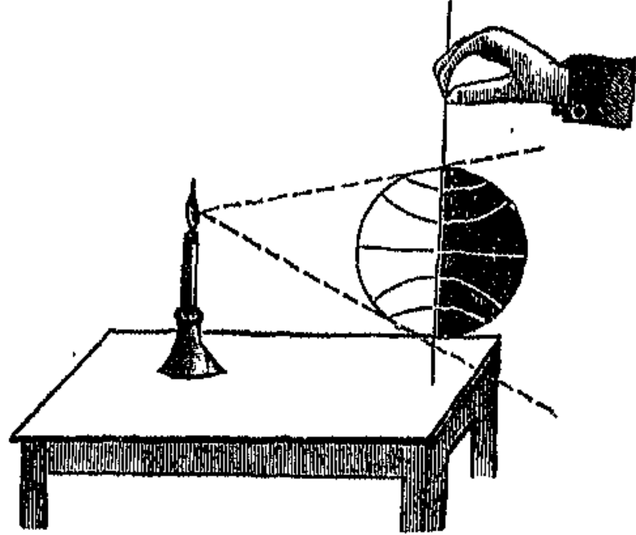
৭৮ চিত্র।—সমান দিন রাত।
