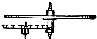
Fig. 43.—Cylinder Escapement
