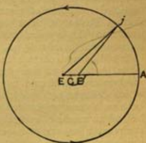
FIG. 35.—The equant.
