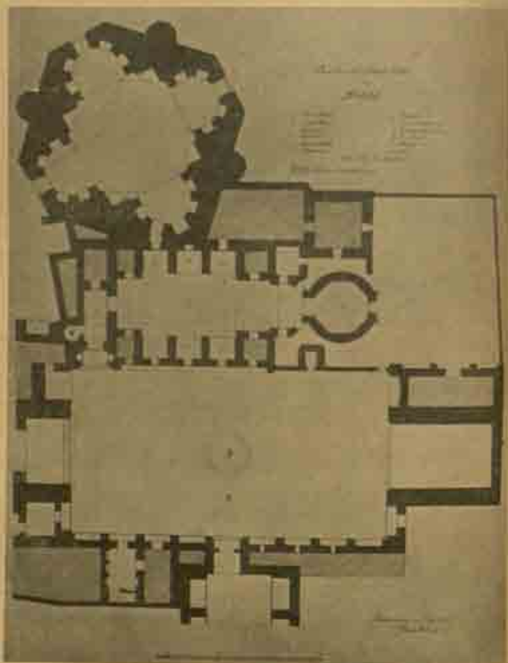
Fig. 285. — Mosquée de Cheikh-Soltan à Ardabil, commencée au x e et achevée terminée sous Chah-Abbas (1612-1627). Plan d'après Reuss-Schultz (Séjour, op. cit.).
