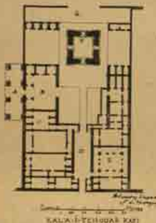
Fig. 12. — Petit palais de Kala-i-Tcheour Kapi à Kase-i-Chirin, dessin de H. Saladin, d'après J. de Morgan.
