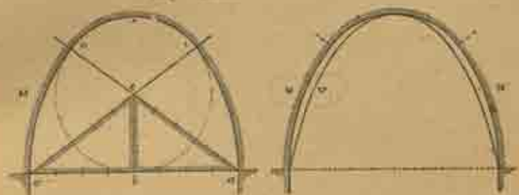
Fig. 8. — Tracé de l'arc égyptien et de l'arc en chaînette d'après A. Choley. — L'art de bâtir chez les Égyptiens.
