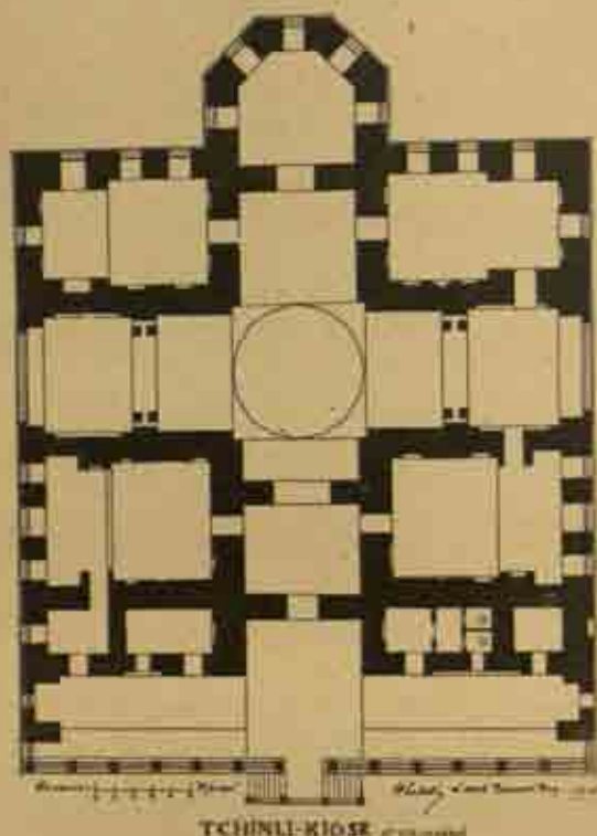
Fig. 300. — Plan du Tchinli-kiosk à Constantinople; commencé en 879 (1496), achevé en 877 H. (1479 J.-C.) par l'architecte Kemal-el-din; restauré en 900 H. (1500 J.-C.) sous le règne du sultan Mémed III.
