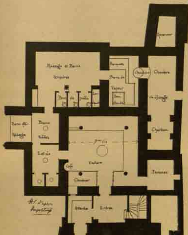
Fig. 225. — Plan des houts du palais du Bardo près de Tunis. — Dessin de H. Saladin, d'après Duperloy.
