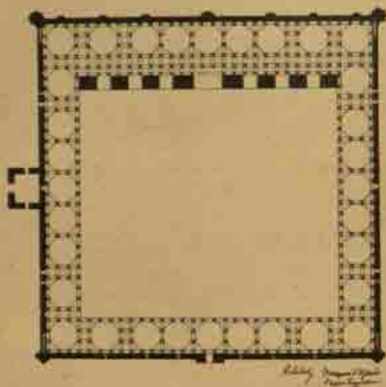
Fig. 306. — Plan de la mosquée d'Ajmer, commencée en 1200, terminée sous Altamach (1211-1236), dessin de H. Saladin, d'après Fergusson.
