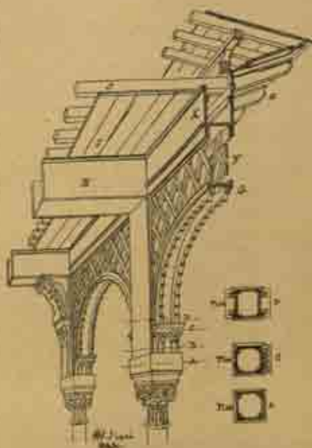
Fig. 186. — Détail de la construction des portiques de l'Alhambra d'après Ulric. — Dessin de H. Saladin.
