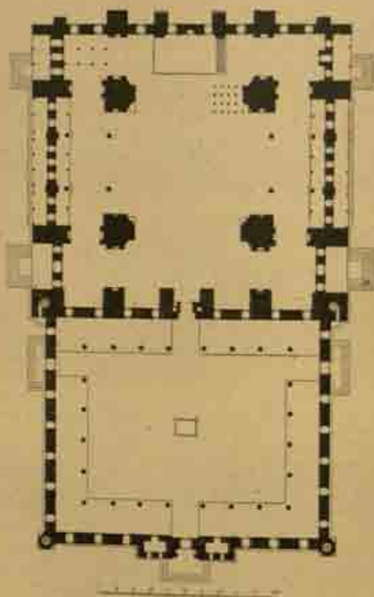
Fig. 371. — Plan de la mosquée Süleymaniye, à Constantinople.
