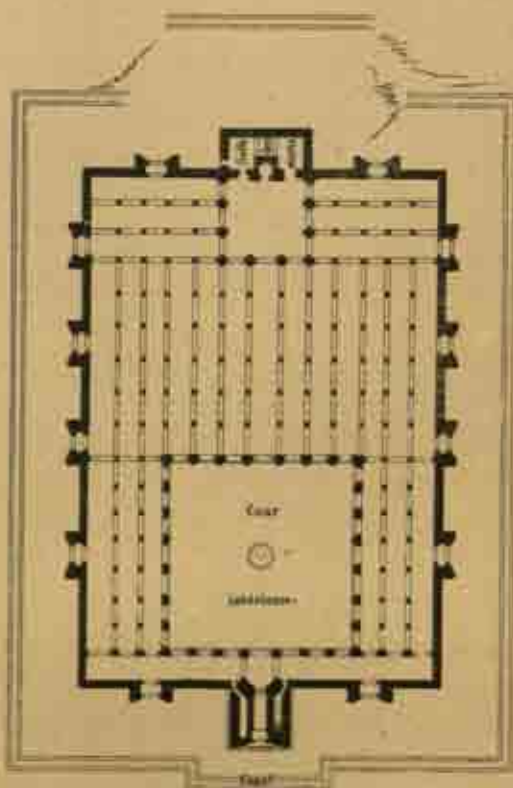
Fig. 186. — Plan de mosquée de Mousourah à Tlemcen, d'après Lafontaine (731-1537 à 741-1543).
