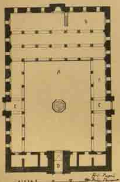
Fig. 47. — Plan de la mosquée Touloun Abou Bezzik au Caire. Dessin de H. Saladin, d'après Perse d'Avenais.
