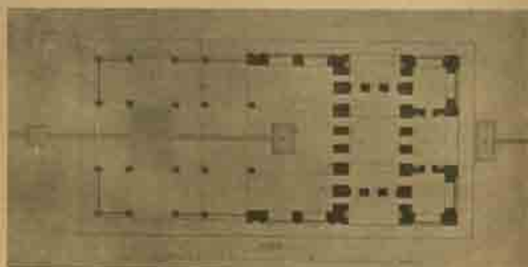
Fig. 413. — Plan du kiosque des miroirs à Isfahan, par Pascal Coste-Alouch-khané 2 .
