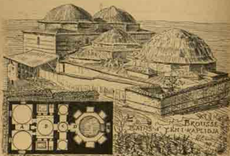
Fig. 367. — Bains de Brouse construits vers 960 H. (1553 J.-C.), restaurés vers 1008 H. (1587 J.-C.). Plan et vue perspective. — Dessin de H. Saladin.
