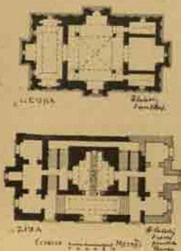
Fig. 152. — Plans de la Cuba et de la Zina, à Palerme. Zina, 493 H—1154 J.-C. — Cuba, 575 H—1180 J.-C. — Dessin de H. Saladin.
