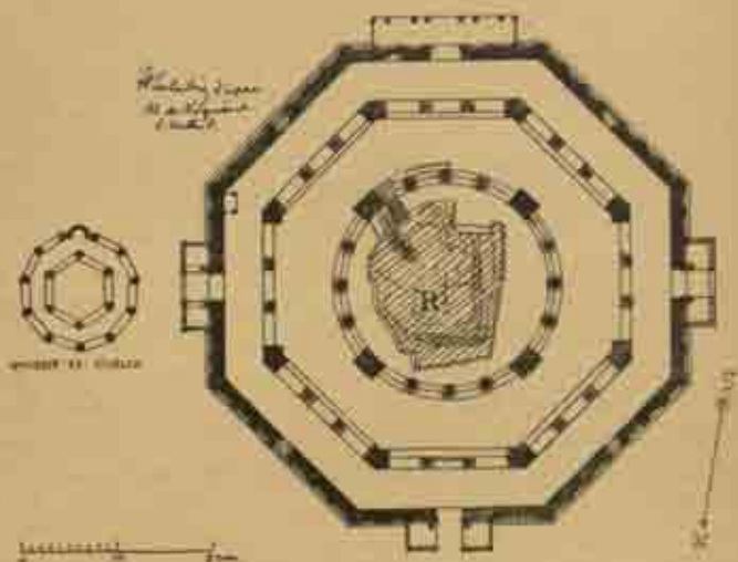
Fig. 22. — Plan de la Koubbet-es-Sakhra (mosquée d'Omar); d'après H. Saladin, d'après M. de Vogüe.
