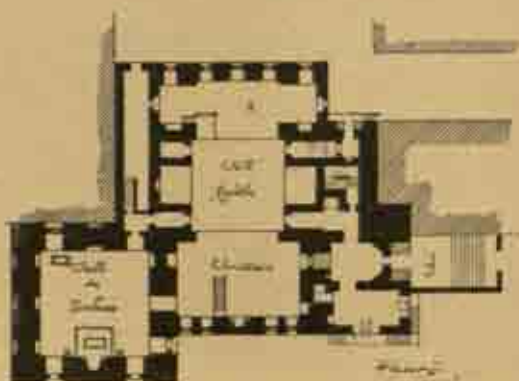
Fig. 97. — Mosquée Kaï-Bey, extra muros au Caire.
