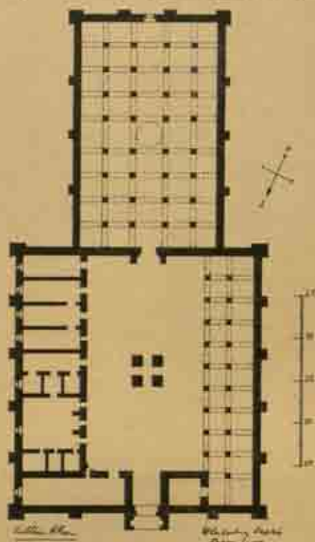
Fig. 342. — Plan du caravansérail de Sultan-Khan (1228-1278).
