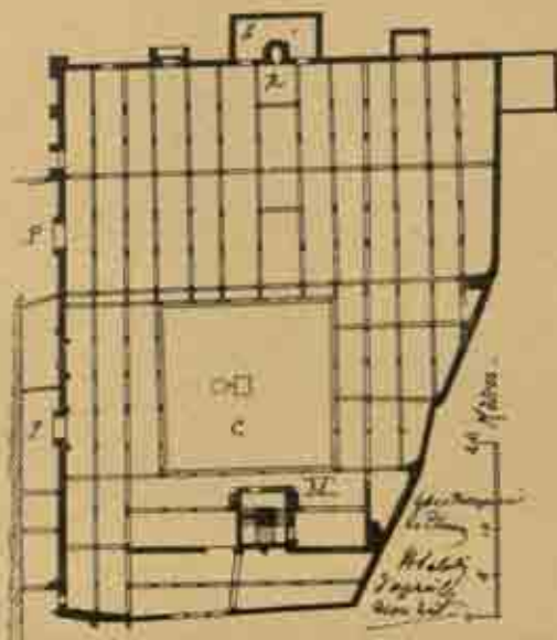
Fig. 143. — Grande mosquée de Tlemcen, dessin de H. Saladin, d'après les archives des Monuments historiques.
