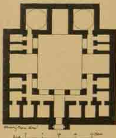
Fig. 341. — Medrassé Ibrahim-bey à Ak-sérail, xi e siècle de l'égire, xiv e de l'ère chrétienne, d'après Sarre. Reise in Kleinasien .
