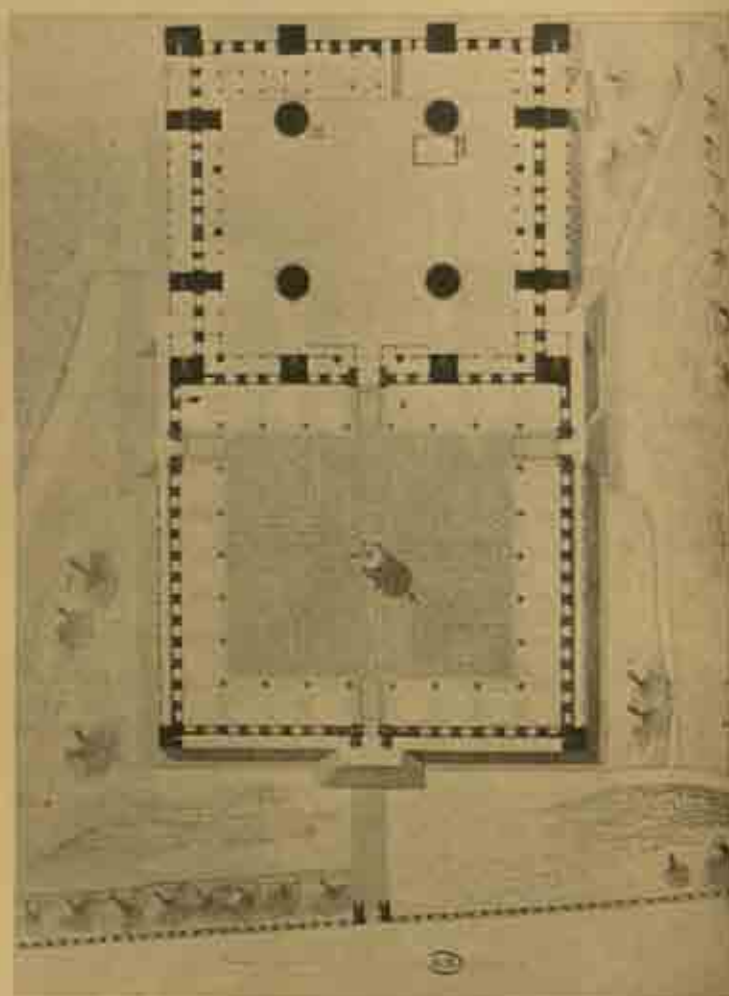
Fig. 385. — Plan de la mosquée du sultan Ahmed I er (1016 H.-1608 à 1023 H.-1615 J.-C.), d'après le relevé de Thomas.
