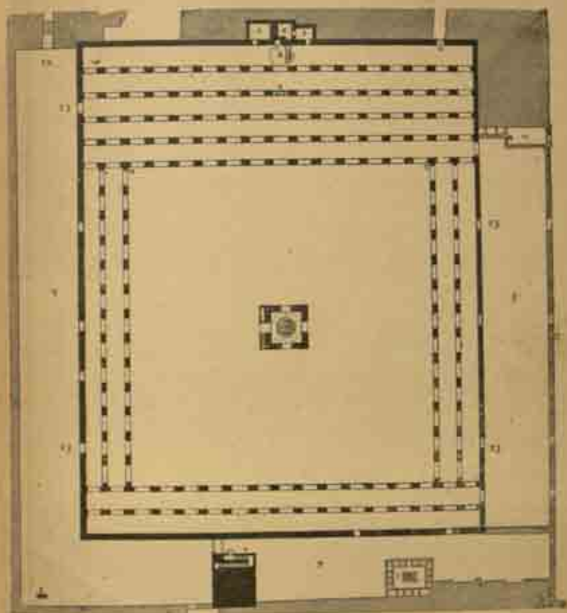
Fig. 11. — Plan de la mosquée d'Elle Trained au Caire. D'après Fournier-Picard.
