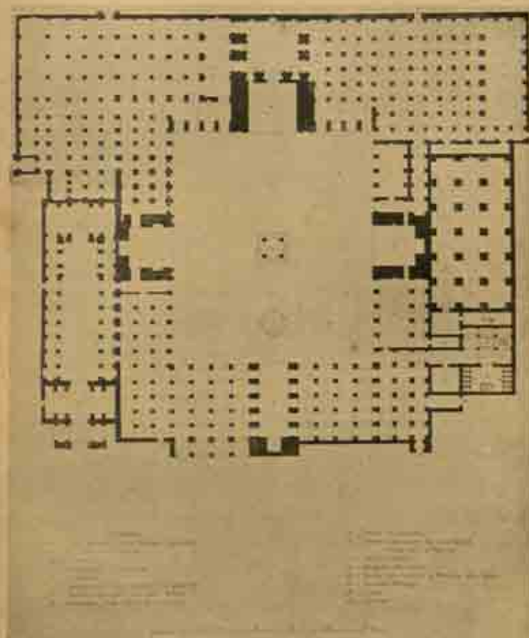
Fig. 254. — Mosquée Djumma à Ispahan — construite de 413 à 452 H. sous le califat de l'abbassade el-Mineour agrandie vers 1080 par Melik Ghâli, réparée sous Ghâh Tamasp (1523-1576) et sous Ghâh Agha (1585-1628). — Plan par P. Coste.
