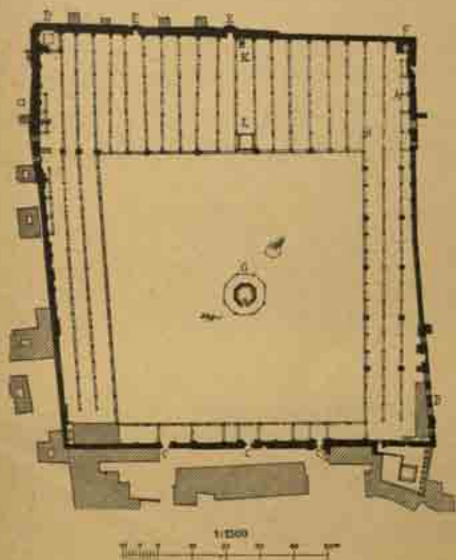
Fig. 29. — Plan de la mosquée d'Auzou au Caire.
