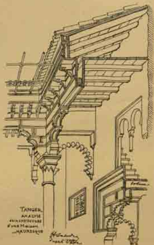
Fig. 225. — Détail de charpente d'une maison à Tanger. — Dessin de H. Saladin, d'après l'Uds. Comparer avec le mode de construction des portiques de l'Alhambra (fig. 196).
