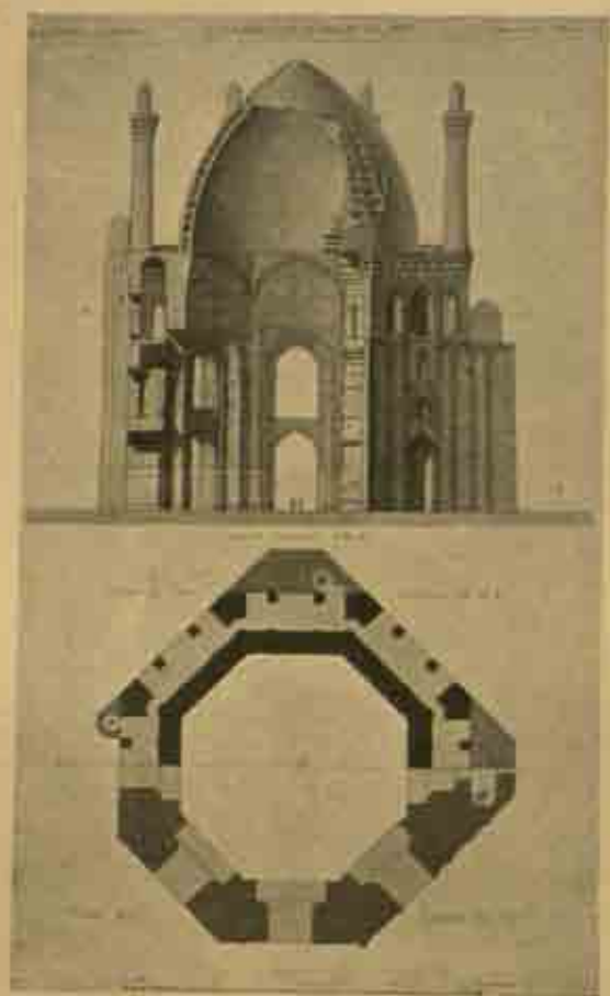
Fig. 266. — Plan et coupe du tombeau d'Ordjahan Khoulahmetli à Sultanich, d'après Dieulafoy (T. II, 1220 J-4).
