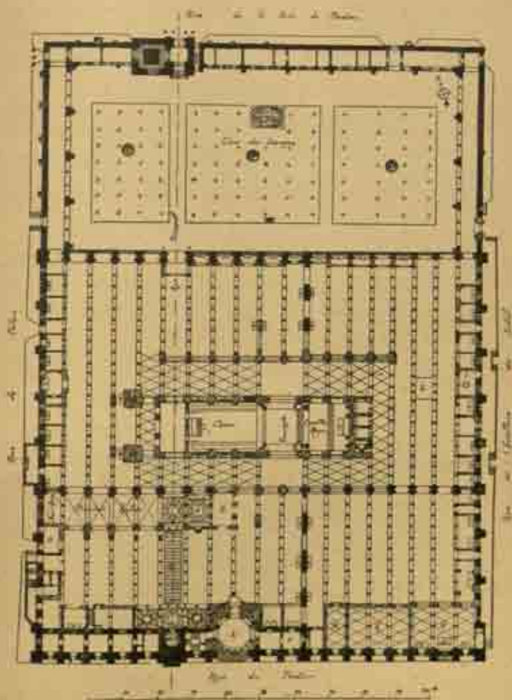
Fig. 139. — Plan de la grande mosquée de Cordoue, d'après Nieu.
