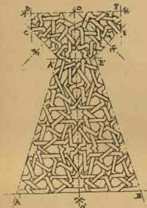
Fig. 267. — Détail d'un huitième du plan d'un plafond en forme de pyramide à exécuter en charpente. — Dessin de H. Saladin, d'après une figure du traité de Diego Lopez de Arenas: Compendio del arte de Carpinteria (Séville, 1602). — DCA'B'E, moitié du plafond octogonal. — A'B' & B', ou des pans du tronc de pyramide. — o o', axe d'une des faces du plafond.
