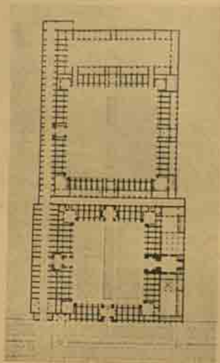
Fig. 367. — Madrasa et caravanserai Madrasa-i-Chah Sultan Husayn à Isfahan (construit en 1506-1510 par Chah Sultan Husayn). — Plan P. Coste.
