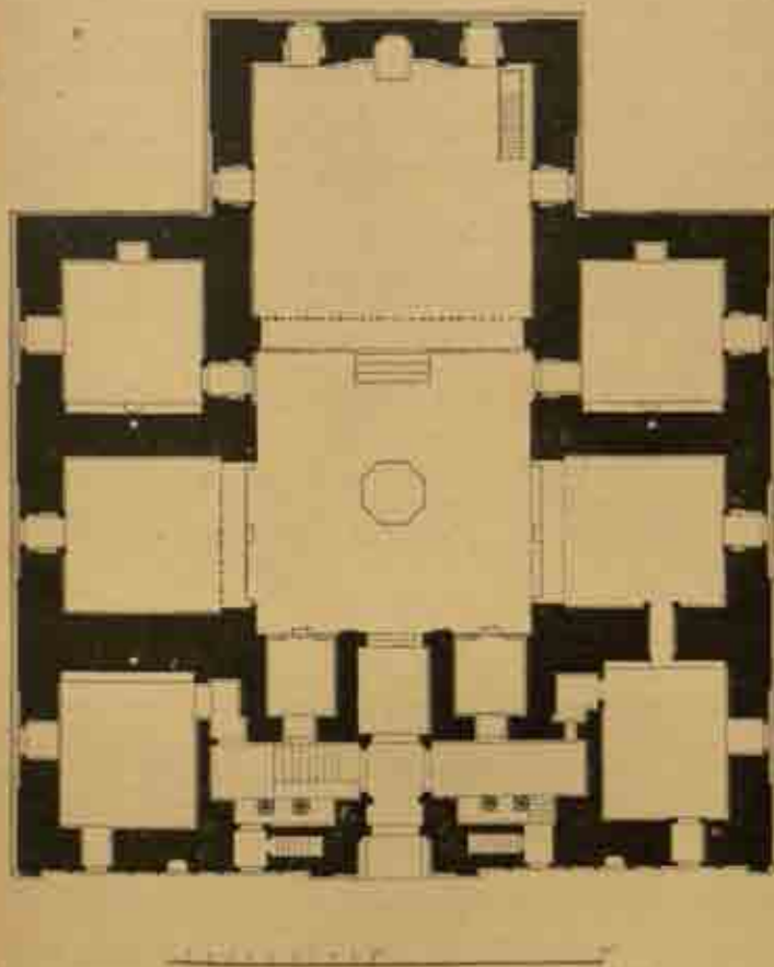
Fig. 366. — Mosquée Verte à Brousse d'après Montan Effendi. Plan du rez-de-chaussée. Du 806 H. (1414 J.-C. à 837 H. (1424 J.-C.).
