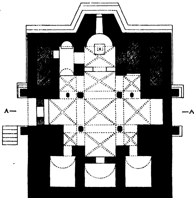
· PLAN OF CRYPT ·
