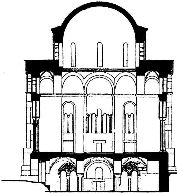
· SECTION ON LINE A-A ·
