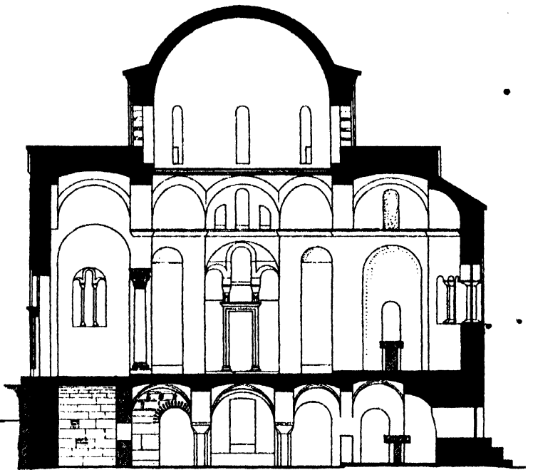
· SECTION ON LINE B-B ·
