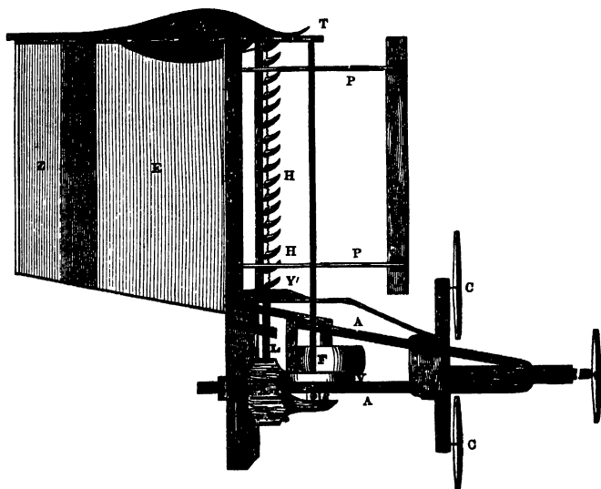
Fig. 26.—Plan.
