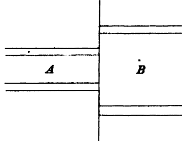
Lateral Shift - Plan.
