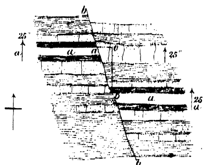
Apparent Lateral Shift - Plan.
