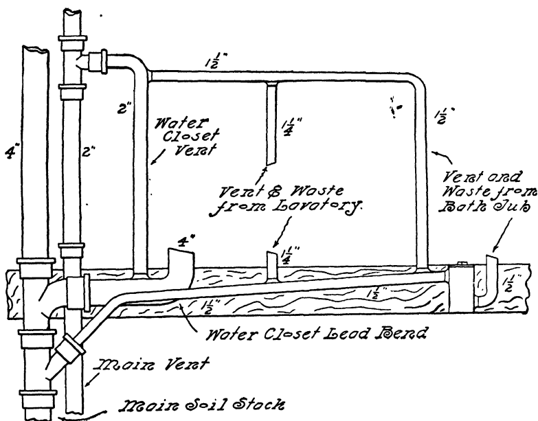
FIG. 90.—“Roughing-in.”
