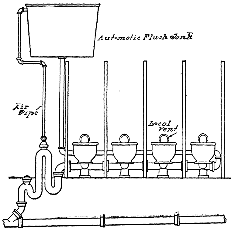
FIG. 160.—Modern Range Water-Closet.
