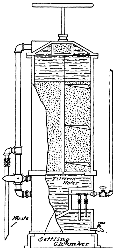
FIG. 232.—Domestic Filter.
