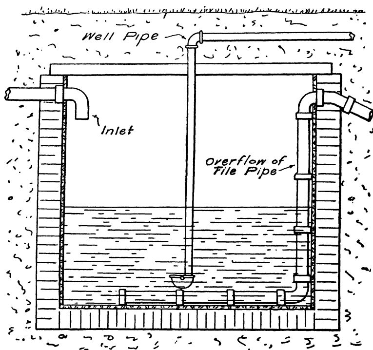
FIG. 246.—Overflow for Cistern.
