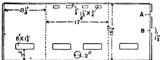
Fig. 217.—Stove Body Pattern.
