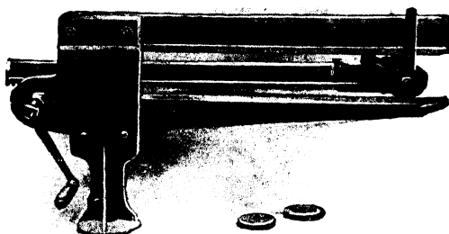
Fig. 59.—Grooving Machine.
