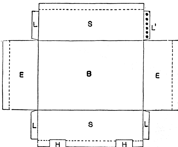
Fig. 71.—Tool Box Pattern.
