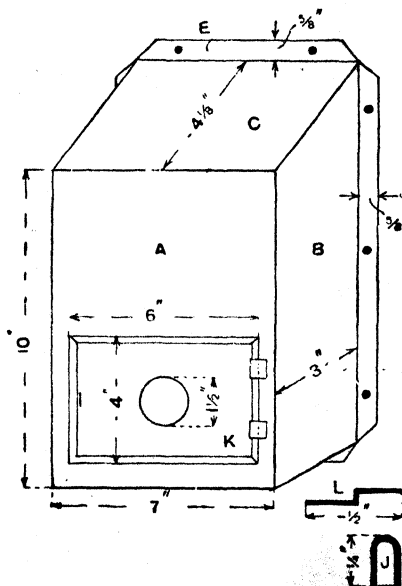
Fig. 84.—Letter Box.
