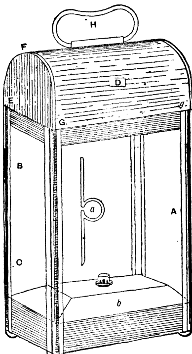
Fig. 250.--Cart Lamp.
