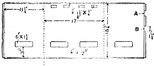
Fig. 217.—Stove Body Pattern.
