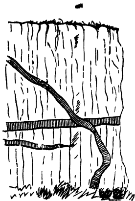
FIG 252 —Basalt Veins traversing bedded dolerites, Kildonan, Ligg
